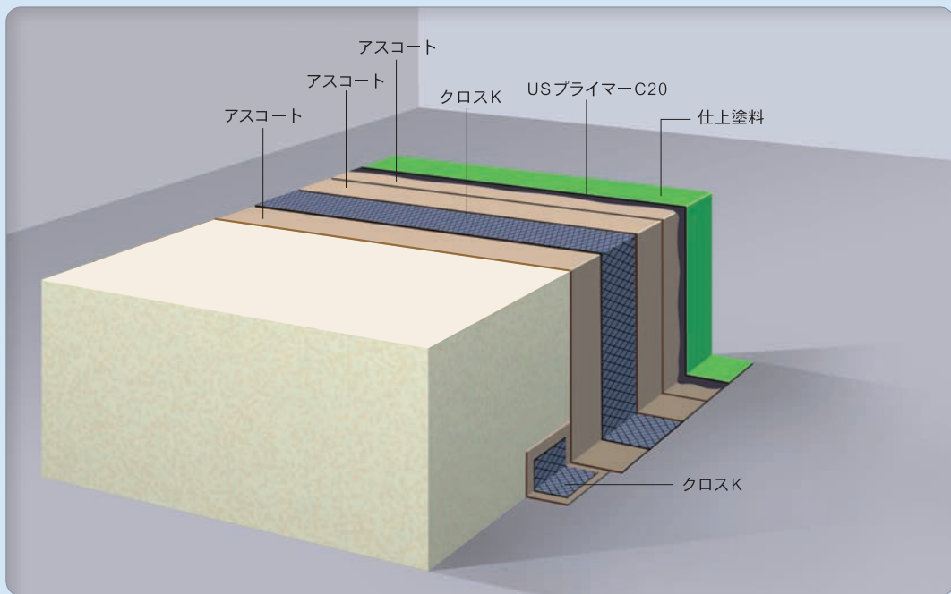
架台回り
