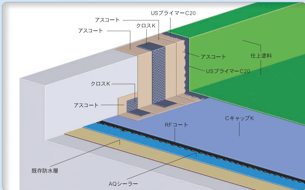
立上り
