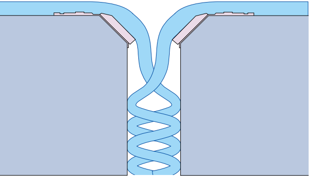
▲ スパイラルドレン
